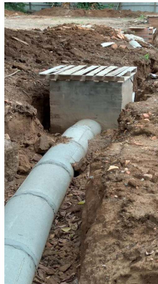
FOTO 10 – Drenagem estacionamento.
