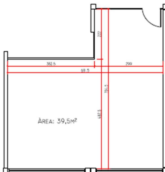
PLANTA BAIXA
